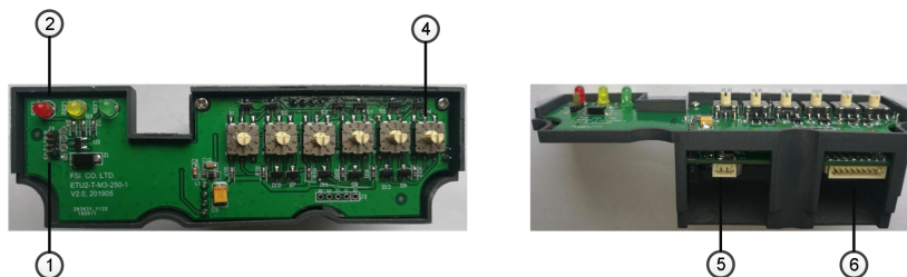
图 2.3 正面图 (M3 系列)
