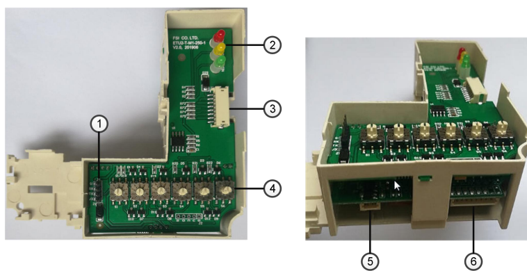
图 2.2 正面图 (M1 系列)
